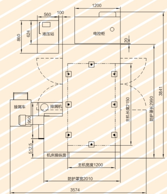
机床平面布置图
